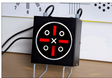
Test de Mallett, dû à la société Gatehouse Industrial Services Ltd.
