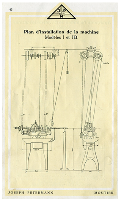
Plan d'installation de la machine modèles 1 et 1B, années 1920. IVR43_20142500914NUC2A
