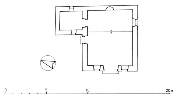
Plan. Dess. Alain Morelière IVR26_20122100526A4YY
