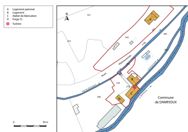
Plan-masse et de situation, section B. Dess. Mathias Papigny IVR43_20142501895NUDA
