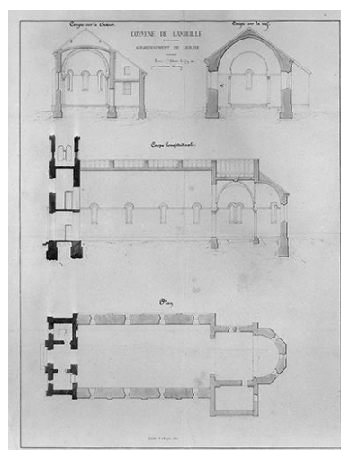
Agrandissement de l'église : plan, coupes longitudinales, sur le chœur et sur la nef, 1864. Phot. Jérôme Mongreville, Phot. Auguste Comoy IVR43_20013900336V
