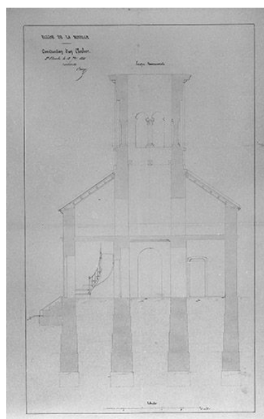
Construction d'un clocher : coupe transversale, 1850. Phot. Jérôme Mongreville, Phot. Auguste Comoy IVR43_20013900327V
