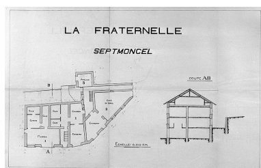
La Fraternelle, Septmoncel [plan du rez-de-chaussée, coupe]. Phot. Jérôme Mongreville, Autr. NEPASUTILISERLecart (ingénieur) IVR43_19963901142X
