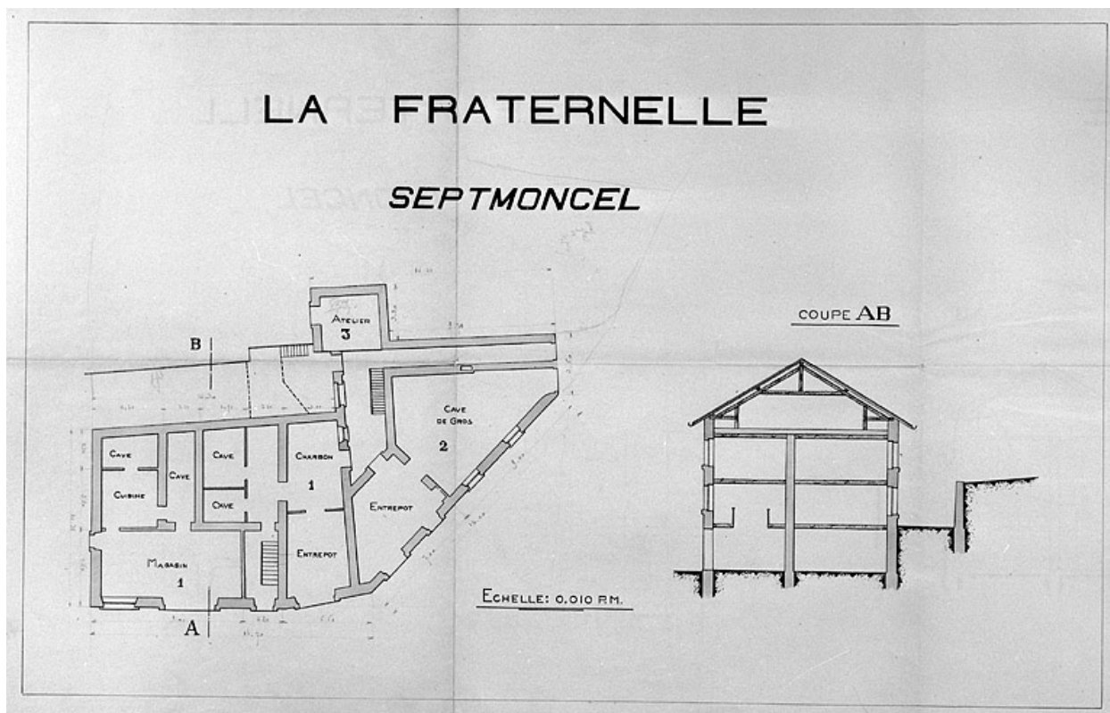
La Fraternelle, Septmoncel [plan du rez-de-chaussée, coupe].
