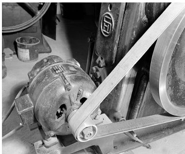
Moteur électrique L. Becquart. Phot. Jérôme Mongreville IVR43_20023900141X
