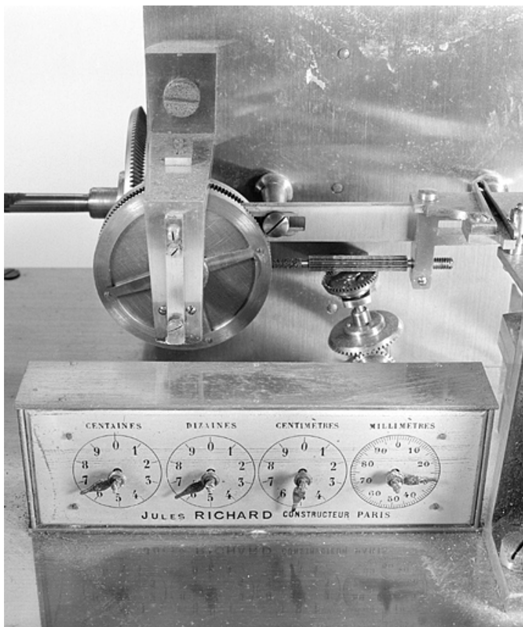
Cadrams et engrenages.
