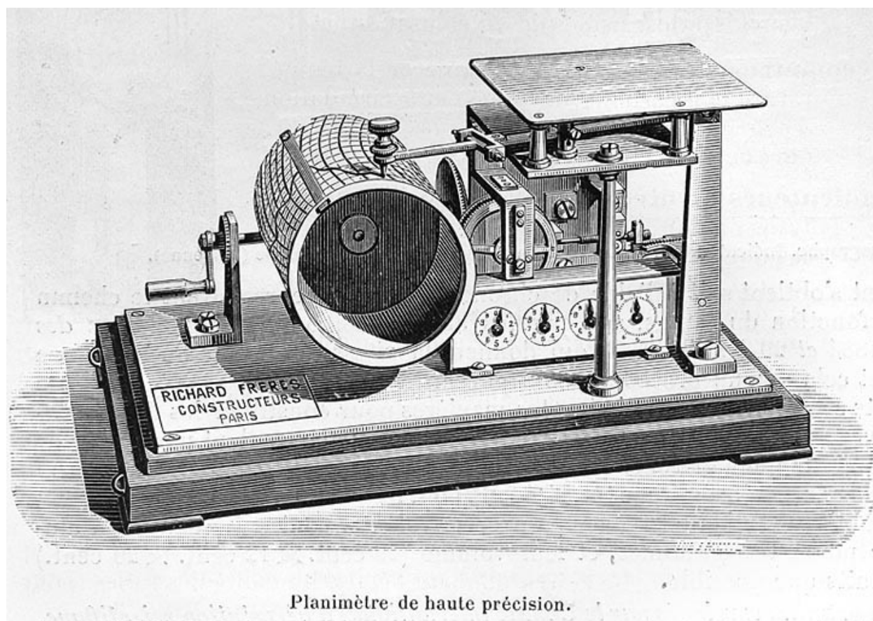
Planimètre de haute précision, 1901.
