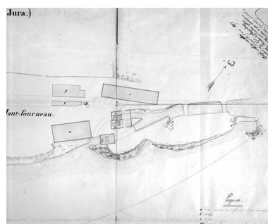
Plan des usines établies sur le Doubs, à Fraisans (Jura) [détail de la Forge Neuve]. Phot. Yves Sancey IVR43_19883900221X
