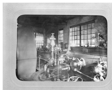
Machine à vapeur Farcot (actionnant le petit train de laminoirs), à la fin du 19e siècle. Phot. Yves Sancey, Phot. De Jongh Frères IVR43_19883900215V
