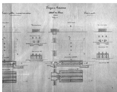
Usine de Fraisans. Détail des fours [les fours à souder]. Phot. Yves Sancey IVR43_19883900225X
