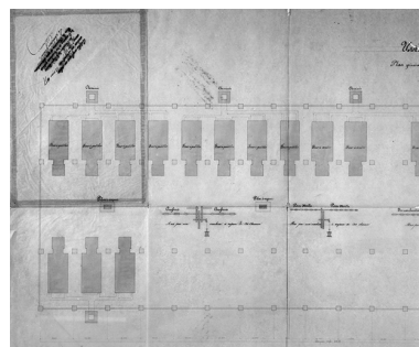
Usine de Fraisans. Plan général de disposition de la Forge [détail de la partie gauche du plan]. Phot. Yves Sancey IVR43_19883900223X
