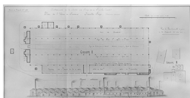
Etablissements de la Société des Forges de Franche-Comté. Plan de l'Usine de Fraisans. Nouvelle Forge. Bâtiment principal. IVR43_19883900227V
