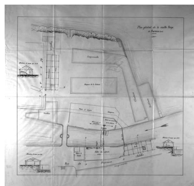
Plan général de la Vieille Forge de Fraisans (Jura). Phot. Yves Sancey IVR43_19883900230V
