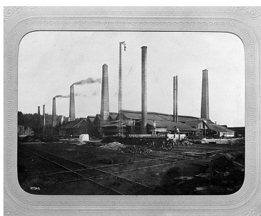
Bâtiment de la Forge Neuve vu du nord, à la fin du 19e siècle. Phot. Yves Sancey, Phot. De Jongh Frères IVR43_19883900213V
