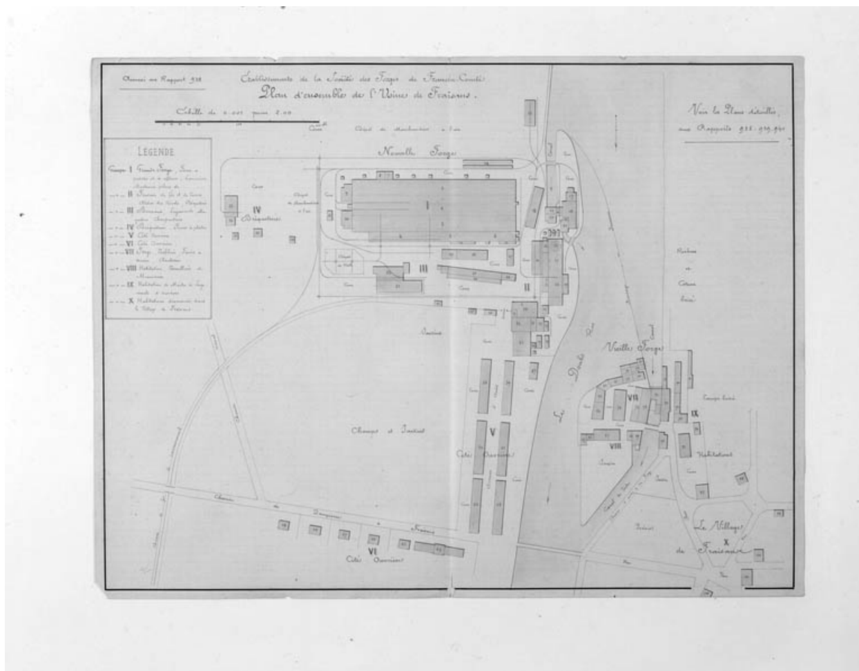
Etablissements de la Société des Forges de Franche-Comté. Plan d'ensemble de l'Usine de Fraisans.
