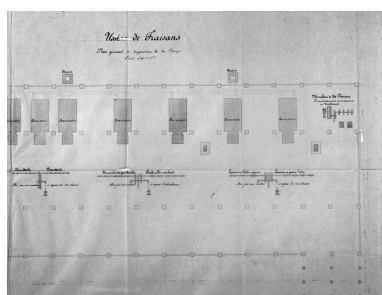
Usine de Fraisans. Plan général de disposition de la Forge [détail de la partie droite du plan]. Phot. Yves Sancey IVR43_19883900224X
