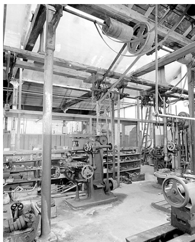
Vue d'ensemble avec le système de transmission. Phot. Yves Sancey IVR43_20022500878X
