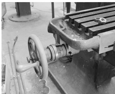
Un des deux volants latéraux avec son disque gradué. Phot. Yves Sancey IVR43_20022500885X
