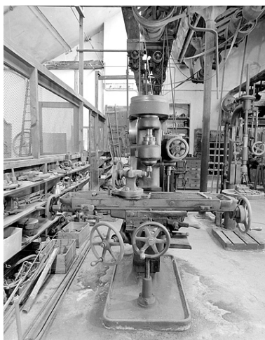
Vue de face. Phot. Yves Sancey IVR43_20022500879X
