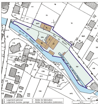
Plan-masse et de situation. Extrait du plan cadastral numérisé, 2005, section AB, 1:1000. Dess. André Céréza IVR43_20067000005NUDA
