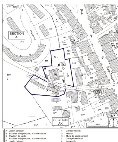
Plan-masse et de situation. Extrait du plan cadastral, 1980, sections AI et AK, échelle 1:1000.
