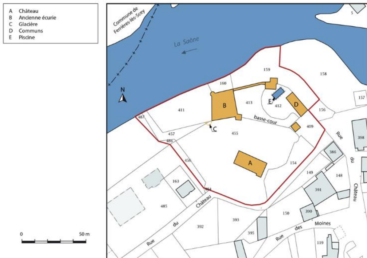
Plan masse de l'ensemble du château et de ses communs
