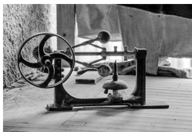
Oscillateur (1979). Phot. J. Dumont IVR43_19792501164Z
