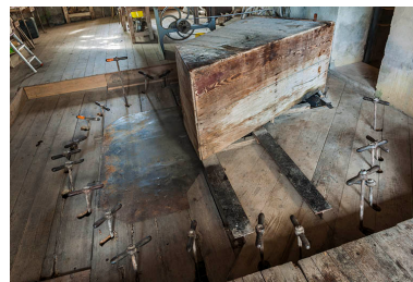
Poignées de commande des pales de la turbine. Phot. Jérôme Mongreville IVR43_20152501883NUC4A
