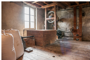
Deuxième étage. Coffre protégeant la transmission mécanique. Phot. Jérôme Mongreville IVR43_20152501872NUC4A
