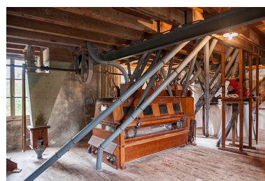
Deuxième étage. Sasseur Nehlig, Heuser et Cie. Phot. Jérôme Mongreville IVR43_20152501870NUC4A
