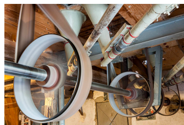
Rez-de-chaussée. Poulies et courroies en mouvement sur l'axe de transmission. Phot. Jérôme Mongreville IVR43_20152501881NUC4A
