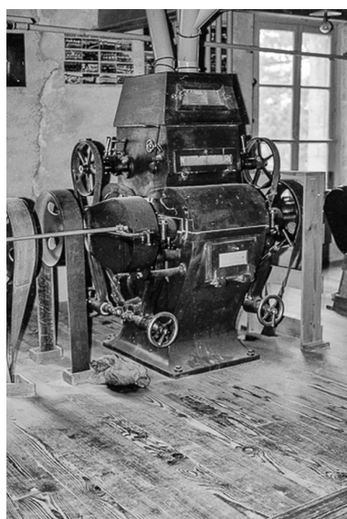
Broyeur à cylindres (1979). Phot. J. Dumont IVR43_19792501165Z
