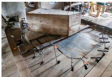
Poignées de commande des pales de la turbine et coffre couvrant la transmission. Phot. Jérôme Mongreville IVR43_20152501885NUC4A
