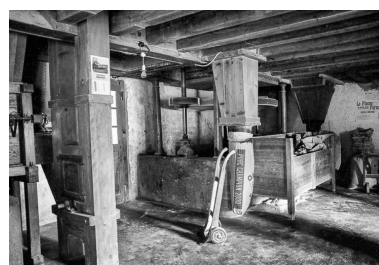
Poste d'ensachage (1979). Phot. J. Dumont IVR43_19792501167Z
