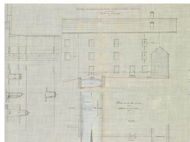
Projet de règlement du moulin du dessous à Esmoulins appartenant au sieur Bouvet [...]. Elévation de la façade est du moulin et plan de la tête d'eau. Phot. Jérôme Mongreville, Autr. Charbonnel IVR43_20097000041NUC2A
