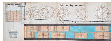
Plan du coursier, s.d. [vers 1860]. Phot. Jérôme Mongreville IVR43_20182500127NUC4A
