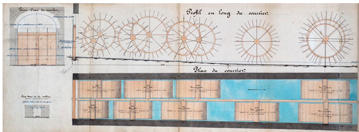
Plan du coursier, s.d. [vers 1860].
