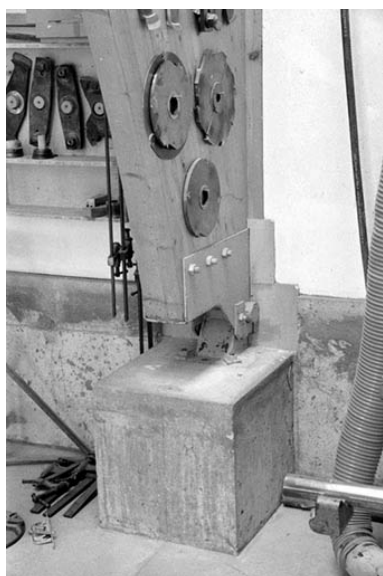
Support d'une ferme de la charpente. Phot. Laurent Poupard IVR43_19883900151Z
