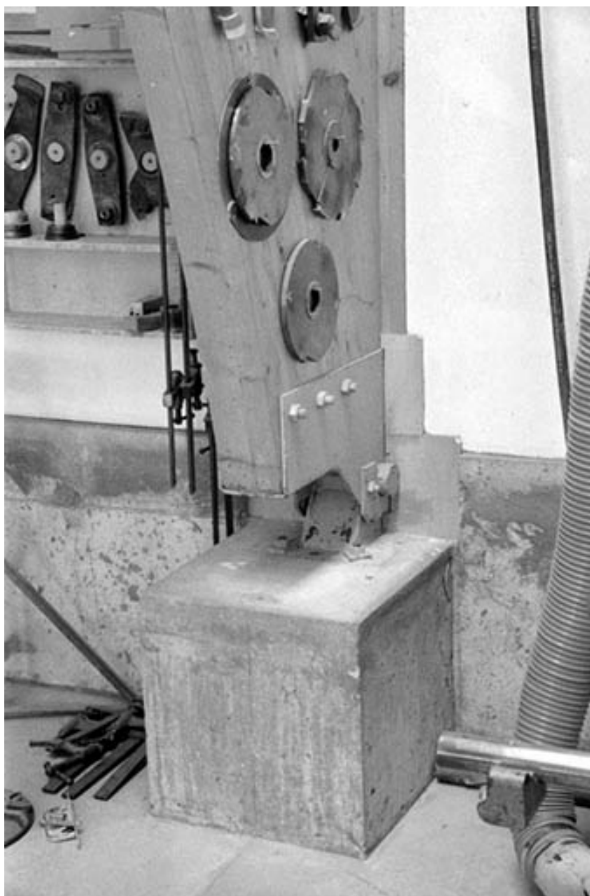
Support d'une ferme de la charpente.
