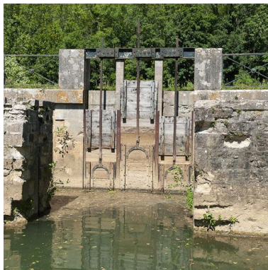
Détail des vannes en bois.
