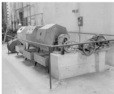
Vue d'ensemble avec le moteur et le réducteur de vitesses. Phot. Jérôme Mongreville IVR43_20022500517X
