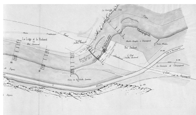
Plan général. Règlement d'eau du barrage de l'usine projetée au lieu-dit "La Roche Lardière" [...]. Phot. Yves Sancey, Phot. Pernot IVR43_19973901974V
