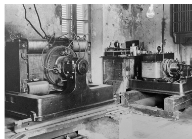
Dynamos de 35 Kw et 15 Kw datant de 1891, 1950-1951. Phot. Yves Sancey, Autr. R. Ponget IVR43_19883900721V
