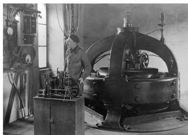
Dynamo de 110 Kw datant de 1891, 1950-1951. Phot. Yves Sancey, Autr. R. Ponget IVR43_19883900722V
