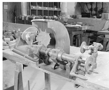
Vue d'ensemble rapprochée de l'arrondisseur (atelier principal). Phot. Jérôme Mongreville IVR43_20022500595X
