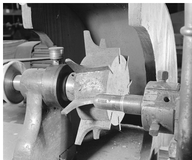
Détail de la fraise et du système de fixation du fourneau par l'intérieur du foyer (arrondisseur de l'atelier principal).
