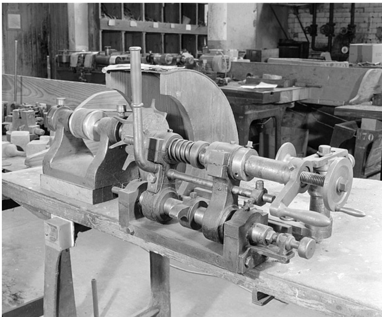
Vue d'ensemble de l'arrondisseur (atelier principal).
