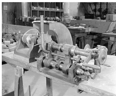
Vue d'ensemble de l'arrondisseur (atelier principal). Phot. Jérôme Mongreville IVR43_20022500594X
