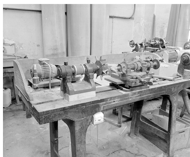
Vue d'ensemble rapprochée de l'arrondisseur (atelier de finissage). Phot. Jérôme Mongreville IVR43_20022500468X
