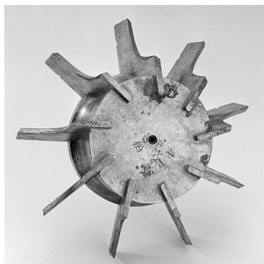
Détail d'une fraise vue de dessus. Phot. Jérôme Mongreville IVR43_20022500953X
