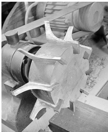
Détail de la fraise (arrondisseur de l'atelier de finissage). Phot. Jérôme Mongreville IVR43_20022500470X
