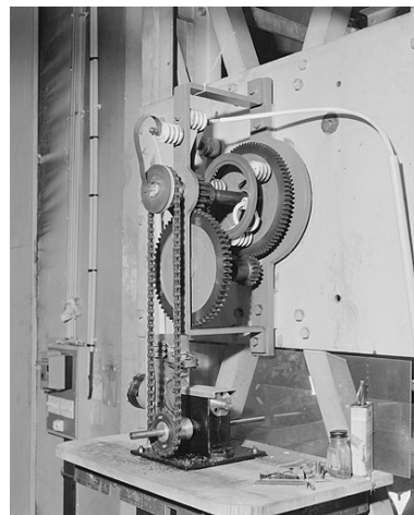
Le système d'entraînement des aiguilles. Phot. Yves Sancey IVR43_20032501151X
