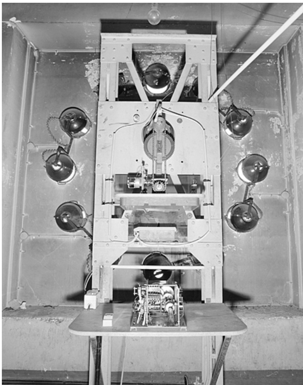
Le mouvement et le cadran, à l'intérieur du bâtiment, de face.
