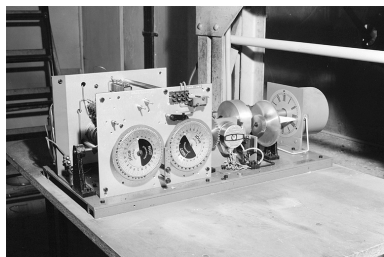
Le mouvement. Phot. Yves Sancey IVR43_20032501149X
