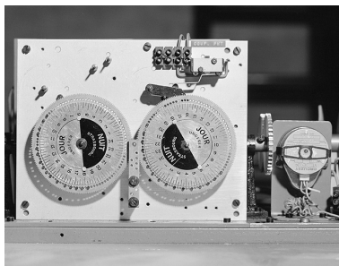
Les cadrans des sonneries. Phot. Yves Sancey IVR43_20032501150X
