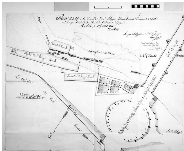
Plan relatif à la demande du Sr Philippe Muneret meunier demeurant à Dôle. Phot. Yves Sancey, Autr. Bietrix IVR43_19903901007X
