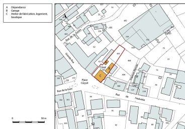
Plan-masse et de situation. Extrait du plan cadastral, 2018, section AA, 1/1 000. Dess. Bertrand Turina IVR43_20182501413NUDA
