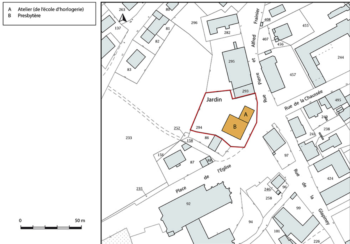
Plan-masse et de situation. Extrait du plan cadastral, 2018, section AB, 1/1 000.
