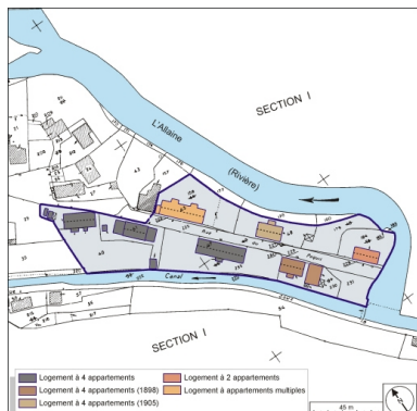
Plan-masse et de situation. Extrait du plan cadastral, 1984, section A, 1:1000 réduit à 1:1500. Dess. André Céréza IVR43_20039000037NUDA
