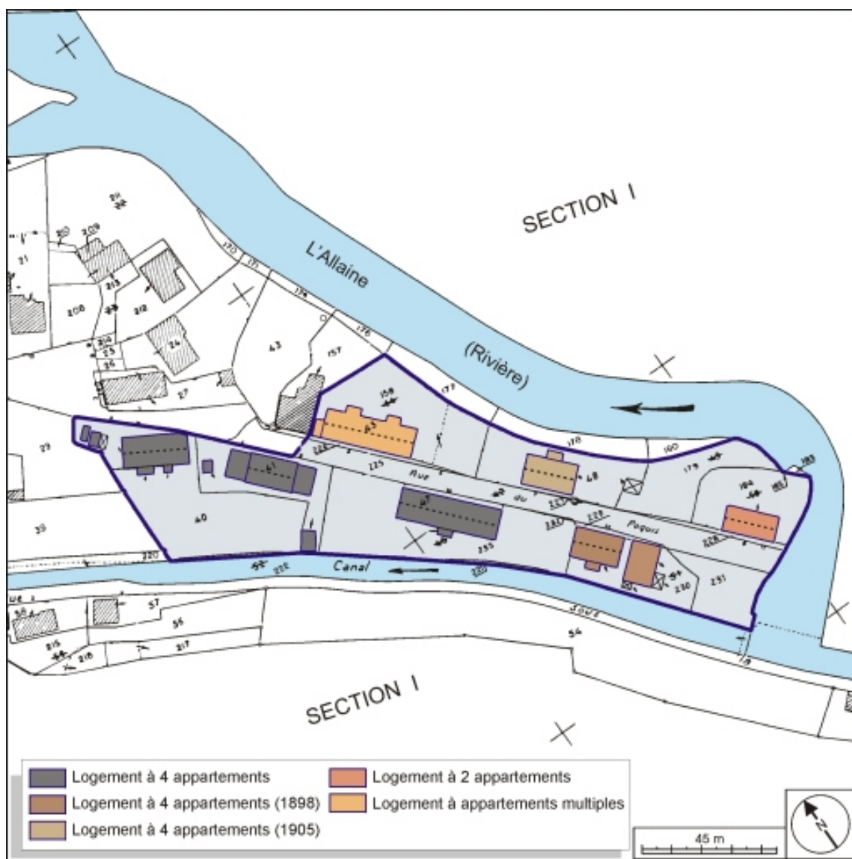
Plan-masse et de situation. Extrait du plan cadastral, 1984, section A, 1:1000 réduit à 1:1500.
