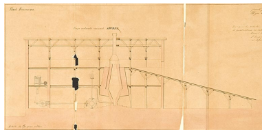
Coupe verticale du bâtiment et du haut fourneau suivant la ligne brisée. Phot. Jérôme Mongreville, Autr. Boudot IVR43_20097000004NUC2A
