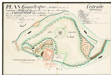
Plan géométrique des usines à fer situées en la commune de Moncey [...], 1828. Phot. Jérôme Mongreville IVR43_20152500587NUC4A
