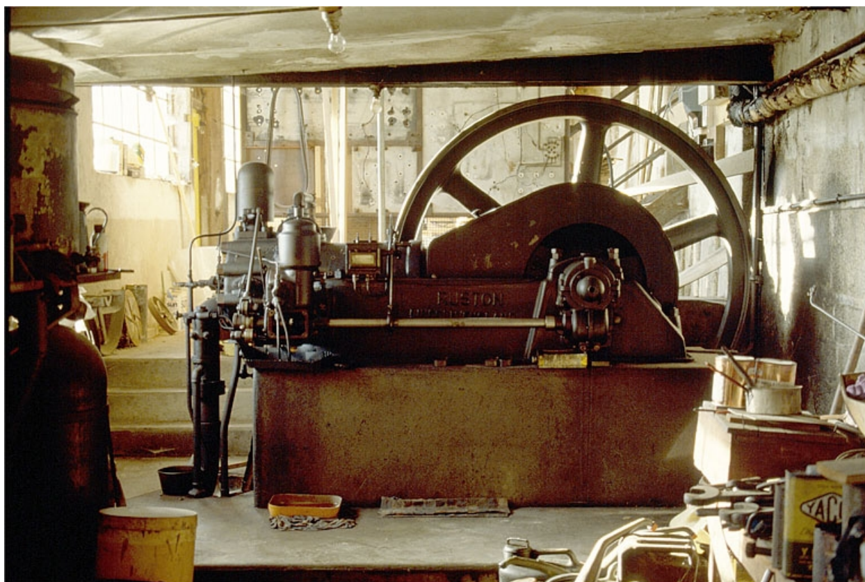
Moteur Ruston et Hornsby. Situé dans le corps de bâtiment en appentis contre la façade postérieure de la minoterie.
