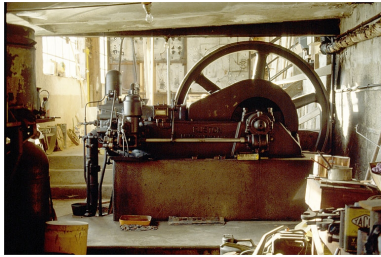
Moteur Ruston et Hornsby. Situé dans le corps de bâtiment en appentis contre la façade postérieure de la minoterie. Phot. Laurent Poupard IVR43_19883900660ZA
