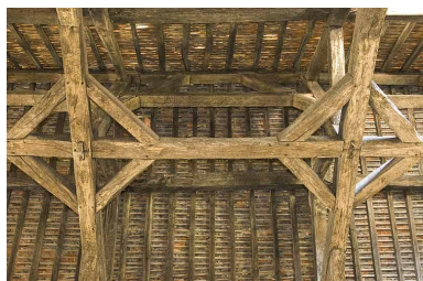
Charpente de la halle à charbon. Travée centrale. Phot. Jérôme Mongreville IVR43_20097000167NUC2A
