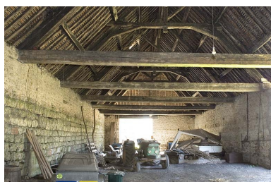
Vue intérieure de la halle à charbon. Partie sud. Phot. Jérôme Mongreville IVR43_20097000169NUC2A
