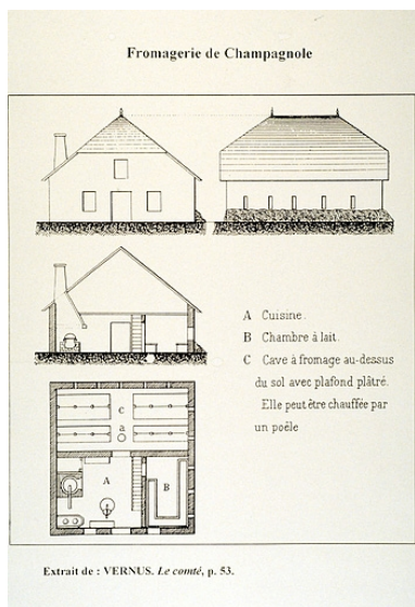
Plan, coupe et élévations du châlet communal. Phot. Jérôme Mongreville IVR43_19953900315ZA
