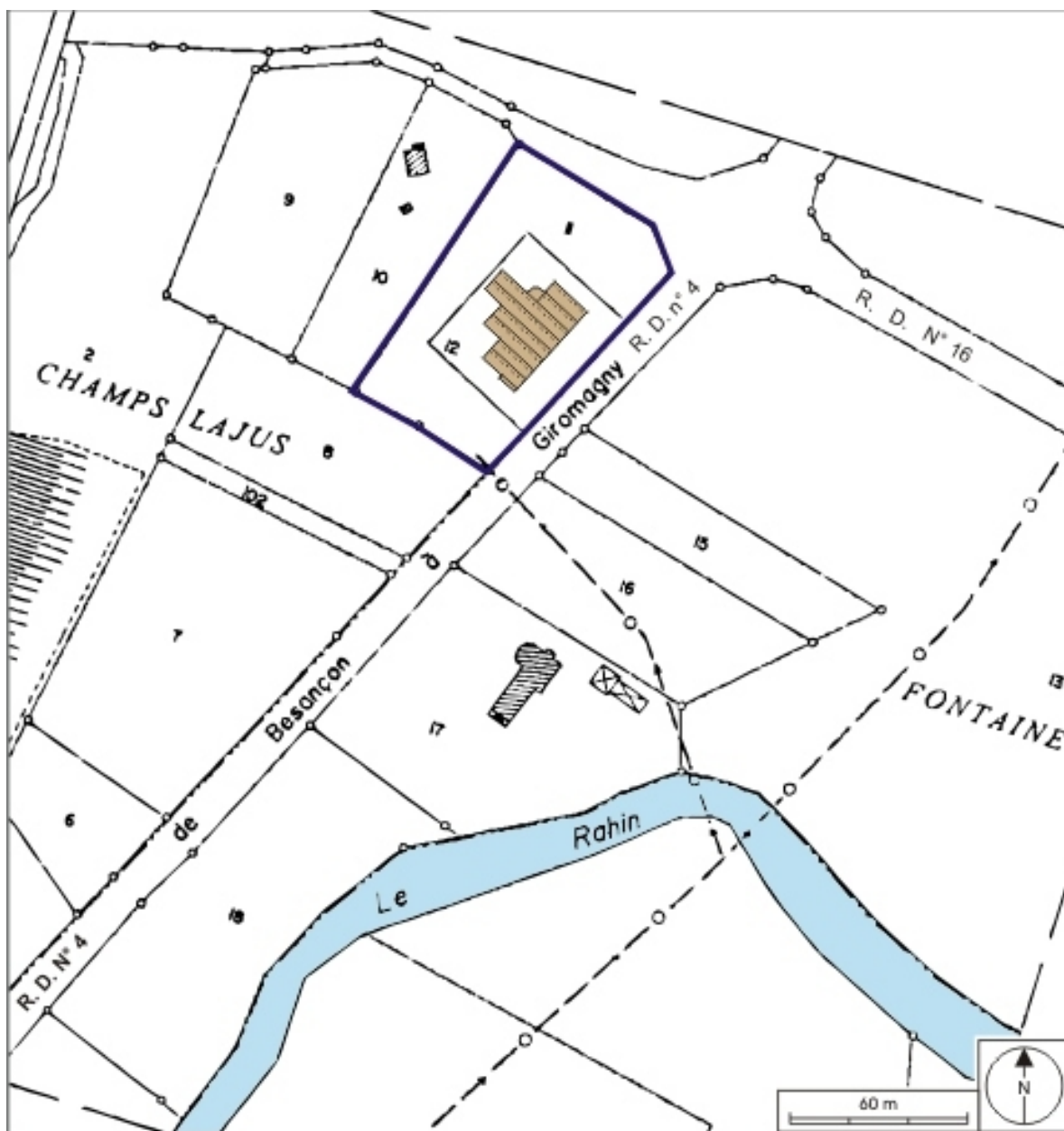
Plan-masse et de situation. Extrait de plan cadastral numérisé, 2008, section ZH, échelle 1:2000. Source : Direction générale des Finances Publiques - Cadastre ; mise à jour : 2008.
