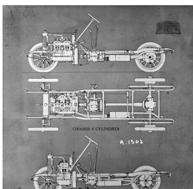
Plan d'un châssis équipé d'un moteur 4 cylindres. IVR43_20122501550NUC2
