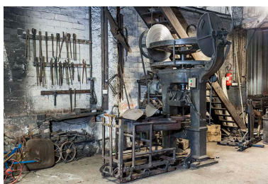
Balancier à friction (emboutissage des socs). Phot. Jérôme Mongreville IVR43_20152501848NUC4A
