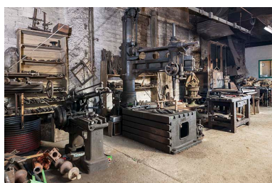
Machines installées contre le mur nord. Vue depuis le sud-ouest. Phot. Jérôme Mongreville IVR43_20152501855NUC4A
