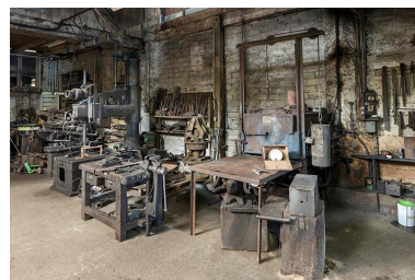
Machines installées contre le mur nord. Vue depuis le sud-est. Phot. Jérôme Mongreville IVR43_20152501862NUC4A
