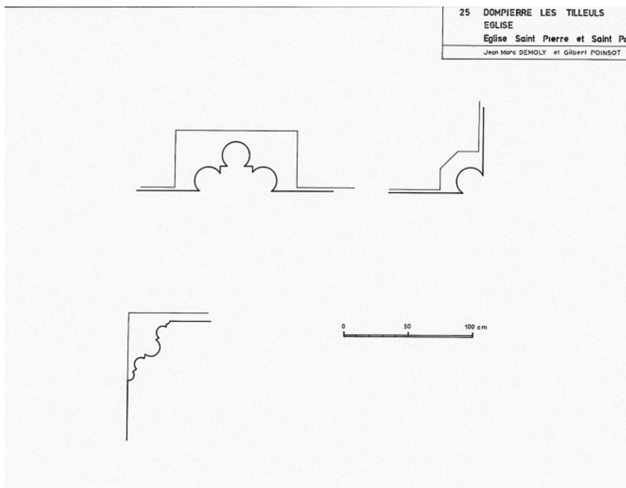
Détail : coupe des colonnes.
