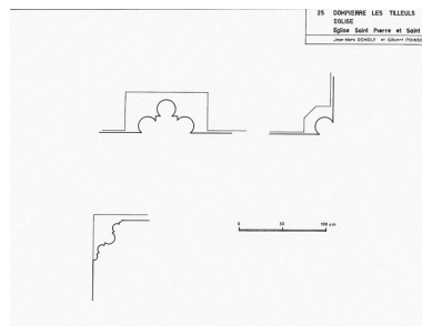
Détail : coupe des colonnes. Phot. Dominique et Sancey Dominguez IVR43_19792500007V
