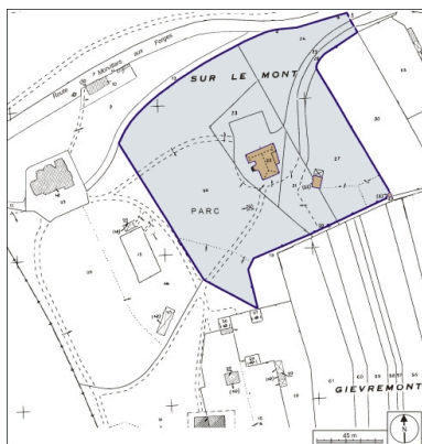
Plan-masse et de situation. Extrait du plan cadastral, 1984, section B, 1:1000 réduit à 1:1500. Dess. André Céréza IVR43_20039000035NUDA
