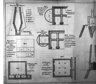
Croquis des appareils situés au gueulard du haut fourneau. Phot. Yves Sancey IVR43_19907000129X
