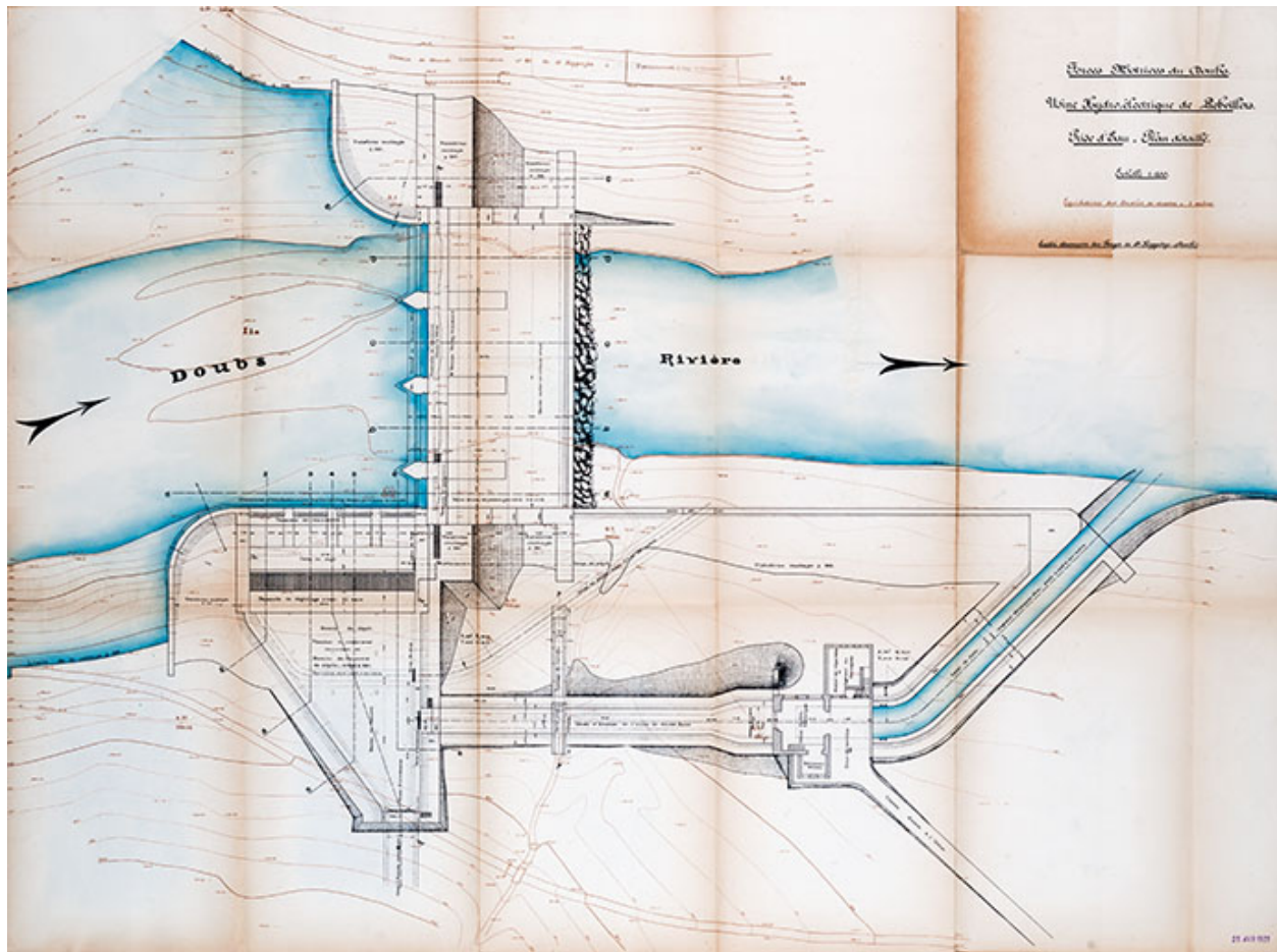
Forces motrices du Doubs. Usine Hydro-Électrique de Liebvillers. Prise d'eau. Plan détaillé, 25 avril 1921.
