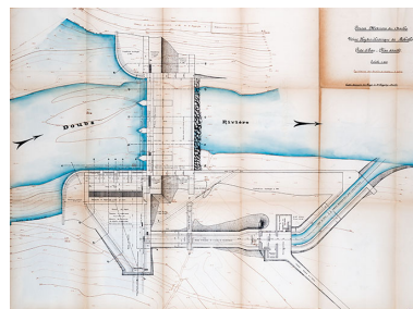
Forces motrices du Doubs. Usine Hydro-Électrique de Liebwillers. Prise d'eau. Plan détaillé, 25 avril 1921. Phot. Jérôme Mongreville, Autr. Émile Andrié IVR43_20132500544NUC4A
