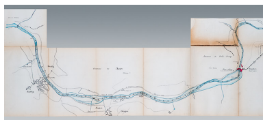
Forces motrices du Doubs. Usine Hydro-Électrique de Liebwillers. Plan sommaire des lieux et des ouvrages projetés [détail de la partie gauche : de Vaufrey à Grosbois], 1er novembre 1920. Phot. Jérôme Mongreville, Autr. Émile Andrié IVR43_20132500552NUC4A
