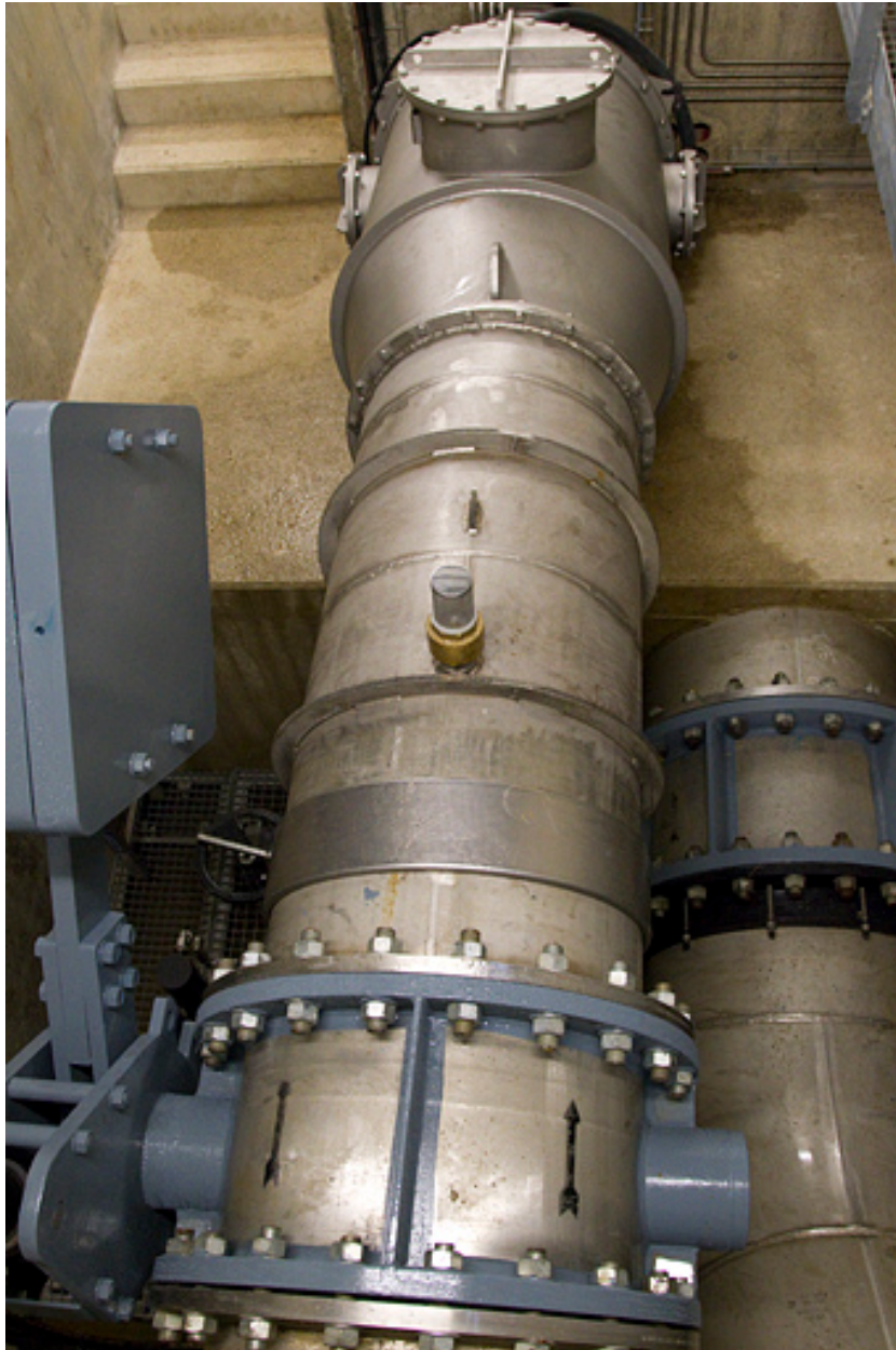
Centrale : nouveau groupe de restitution (vue plongeante).
