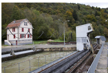
Prise d'eau : vue d'ensemble du dégrilleur. Phot. Yves Sancey IVR43_20122501980NUC2A
