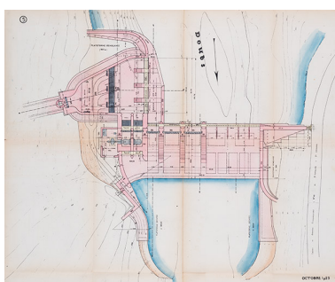
Forces motrices du Doubs. Usine hydro-électrique de Liebwillers [...] Ouvrages amont. Plan d'ensemble, octobre 1923. Phot. Jérôme Mongreville, Autr. auteur inconnu IVR43_20132500559NUC4A
