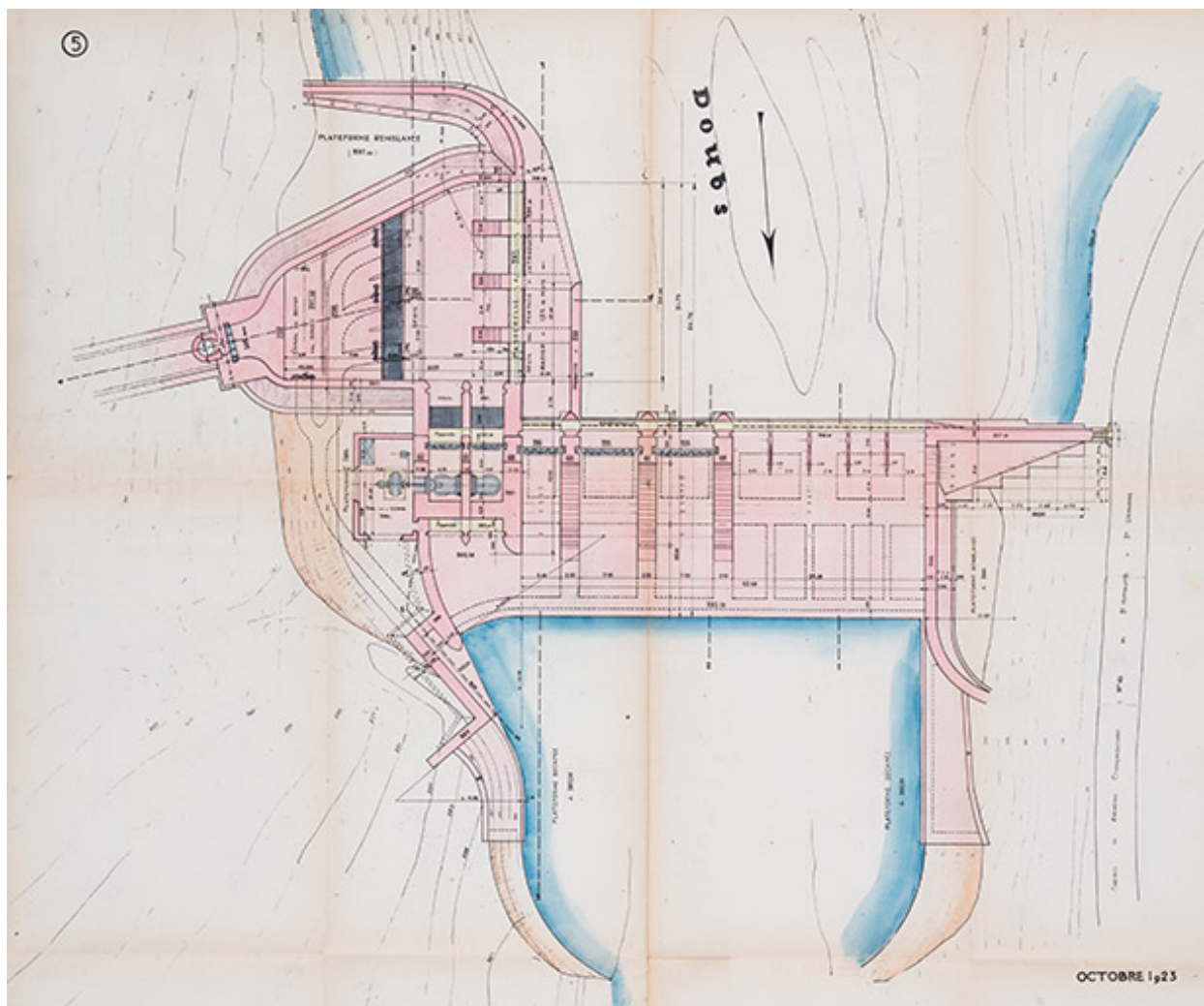
Forces motrices du Doubs. Usine hydro-électrique de Liebvillers [...] Ouvrages amont. Plan d'ensemble, octobre 1923.
