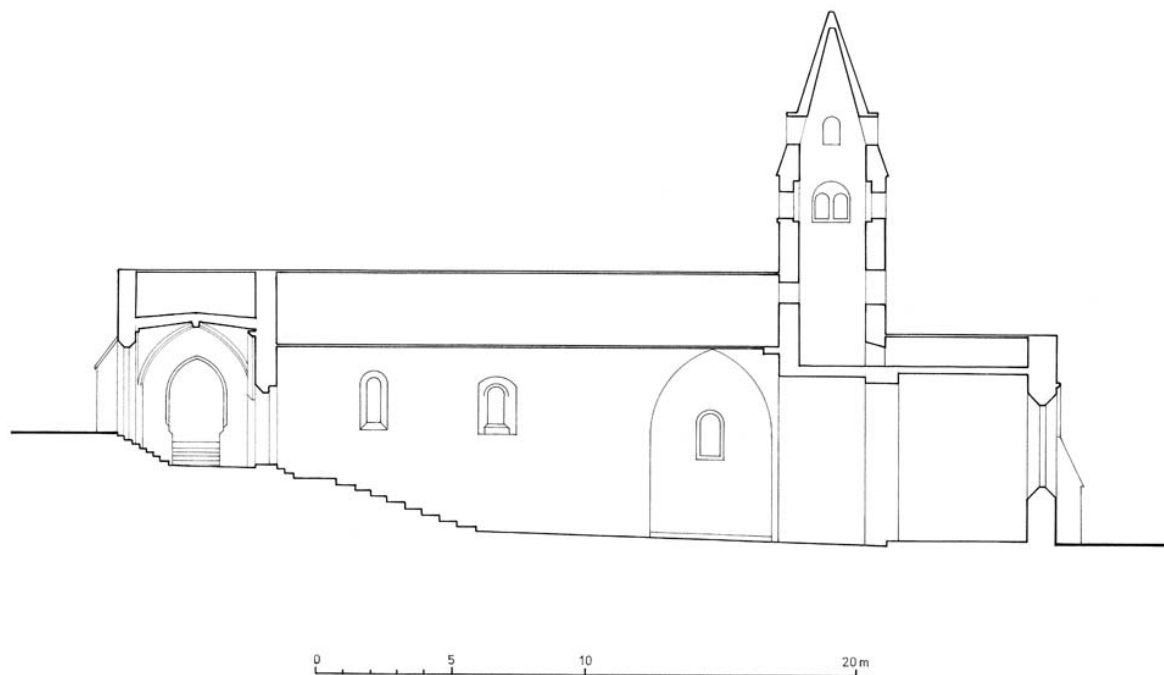
coupe longitudinale
