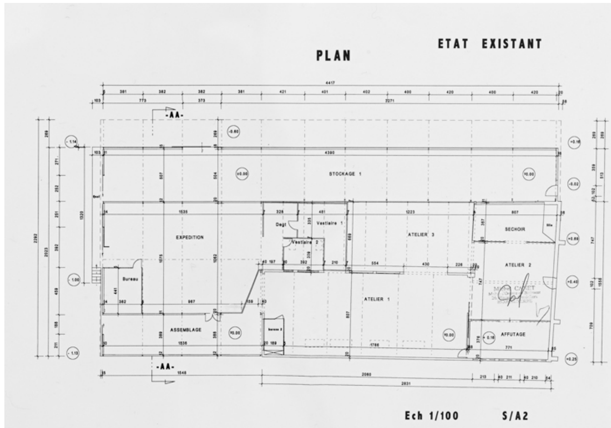
Plan de l'usine de menuiserie en 2004.
