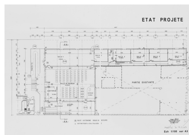
Plan du lieu de culte. Phot. Pierre-Marie Barbe-Richaud, Autr. Michel Canet IVR26_20238901045NUC4A
