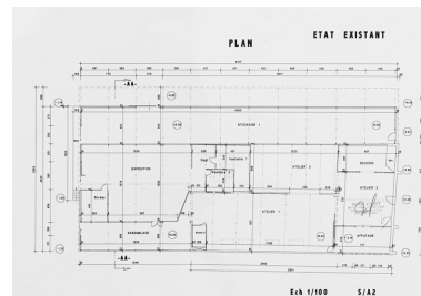
Plan de l'usine de menuiserie en 2004. Phot. Pierre-Marie Barbe- Richaud, Autr. Michel Canet IVR26_20238901039NUC2A
