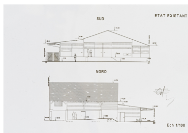
Élévation des façades nord et sud de l'usine de menuiserie. Phot. Pierre-Marie Barbe-Richaud, Autr. Michel Canet IVR26_20238901042NUC2A
