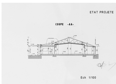
Coupe transversale du lieu de culte évangélique. Phot. Pierre-Marie Barbe-Richaud, Autr. Michel Canet IVR26_20238901043NUC2A
