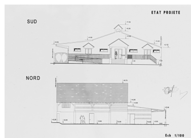
Élévation des façades nord et sud du lieu de culte évangélique. Phot. Pierre-Marie Barbe-Richaud, Autr. Michel Canet IVR26_20238901044NUC2A
