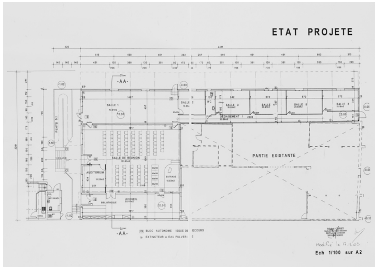
Plan du lieu de culte.
