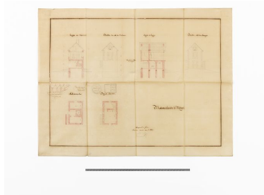
"Maison éclusière de Mingot". Plan, coupe et élévation. (Calque ; 64,5 x 50, Archives VNF- direction territoriale Centre- Bourgogne ; subdivision de Corbigny) Phot. Thierry Kuntz IVR26_20135800010NUC4A
