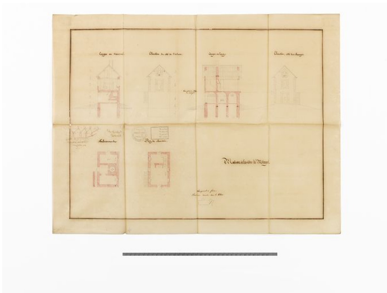
"Maison éclusière de Mingot". Plan, coupe et élévation. (Calque ; 64,5 x 50, Archives VNF-direction territoriale Centre-Bourgogne ; subdivision de Corbigny)
