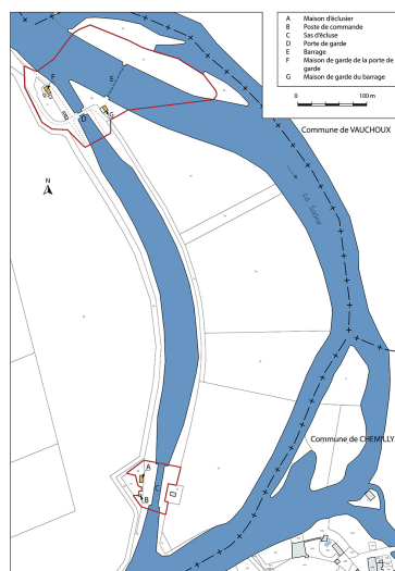
Plan masse et de situation. Détail sud du bief incluant porte de garde et site d'écluse aval.
