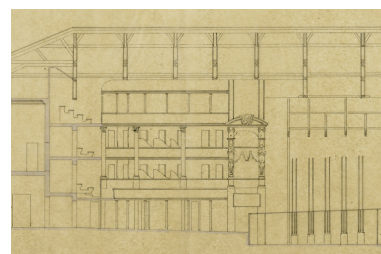
Projet de restauration de la salle de spectacle de la ville de Nevers. Coupe longitudinale [détail de la salle]. 9 avril 1851. Phot. Pierre-Marie Barbe-Richaud, Autr. Hippolyte Paillard IVR26_20245800459NUC4A
