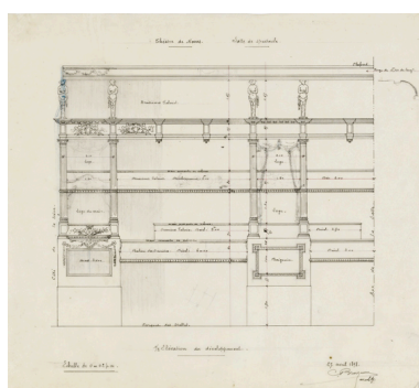
Théâtre de Nevers. Salle de spectacle. 1/2 Elévation du développement. 27 avril 1898. Phot. Pierre-Marie Barbe-Richaud, Autr. Charles Brazeau IVR26_20245800440NUC2A
