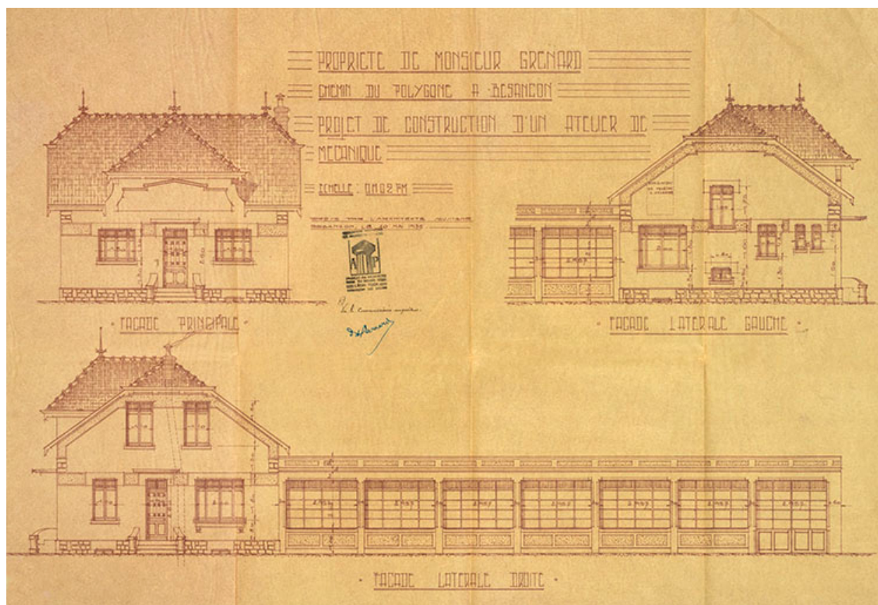
Projet de construction d'un atelier de mécanique [élévation des façades], 1935.
