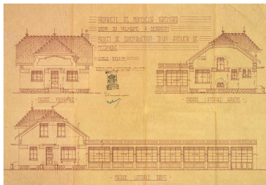
Projet de construction d'un atelier de mécanique [élévation des façades], 1935. IVR43_20192500043NUC4A
