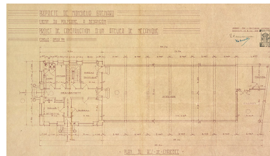
Projet de construction d'un atelier de mécanique [plan du rez-de-chaussée], 1935. IVR43_20192500044NUC4A
