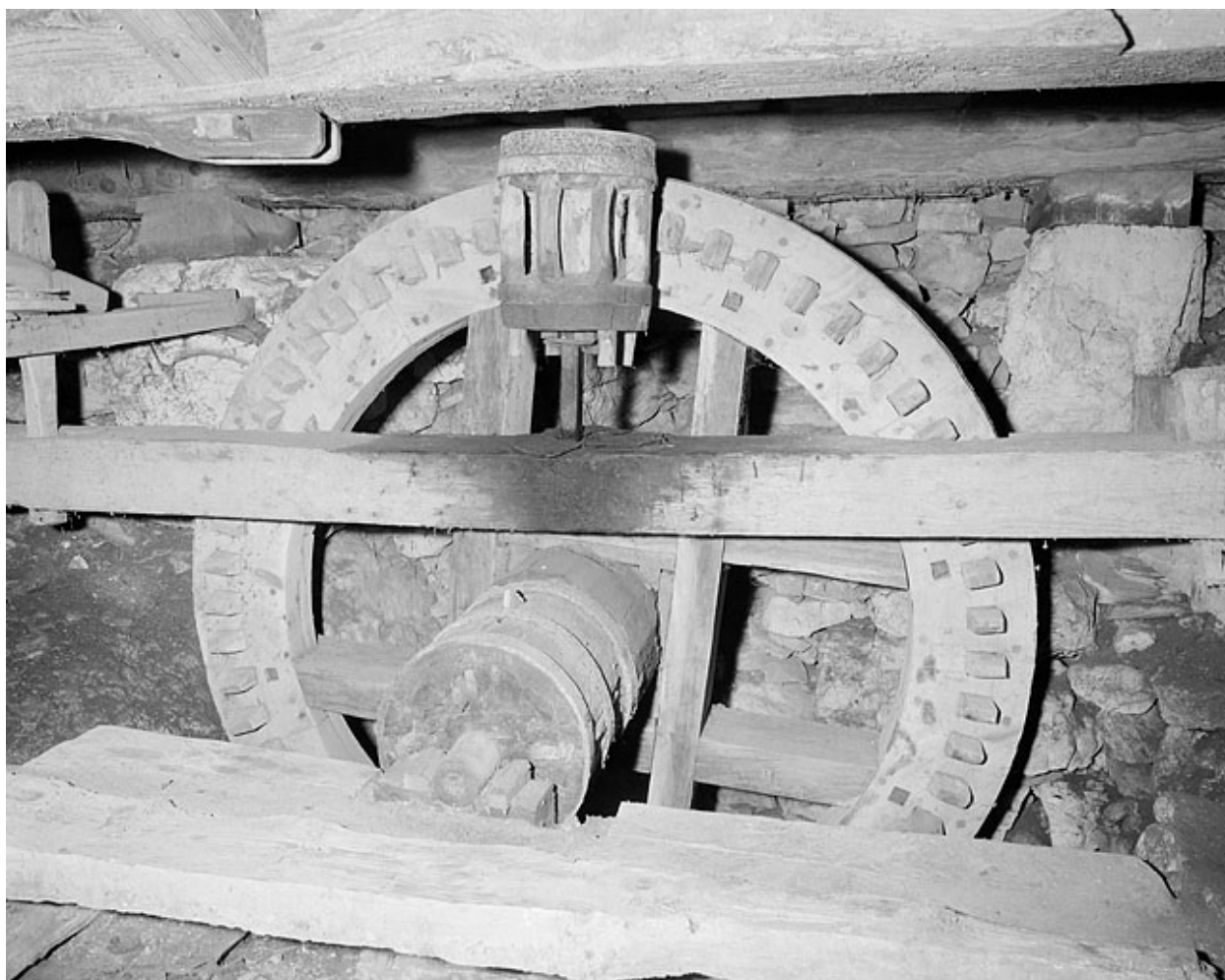
Rouet et lanterne en liaison avec la meule.
