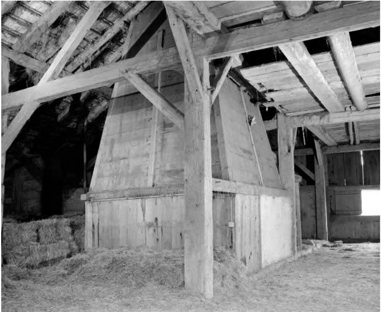
Intérieur : grange et conduit du "tué".
