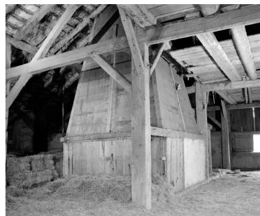
Intérieur : grange et conduit du "tué". Phot. Yves Sancey IVR43_19772500421X
