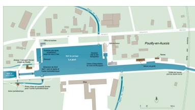
Plan schématique du port de Pouilly-en-Auxois. Dess. Alain Morelière IVR26_20132100096NUDA
