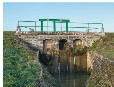
Vue du déversoir. Phot. Pierre-Marie Barbe-Richaud IVR26_20132101046NUC4AQ
