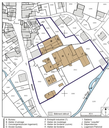
Plan-masse et de situation. Extrait du plan cadastral numérisé, 2008, section B, 1:1250. Source : Direction générale des Finances Publiques - Cadastre ; mise à jour : 2008. Dess. André Céréza IVR43_20087000193NUDA
