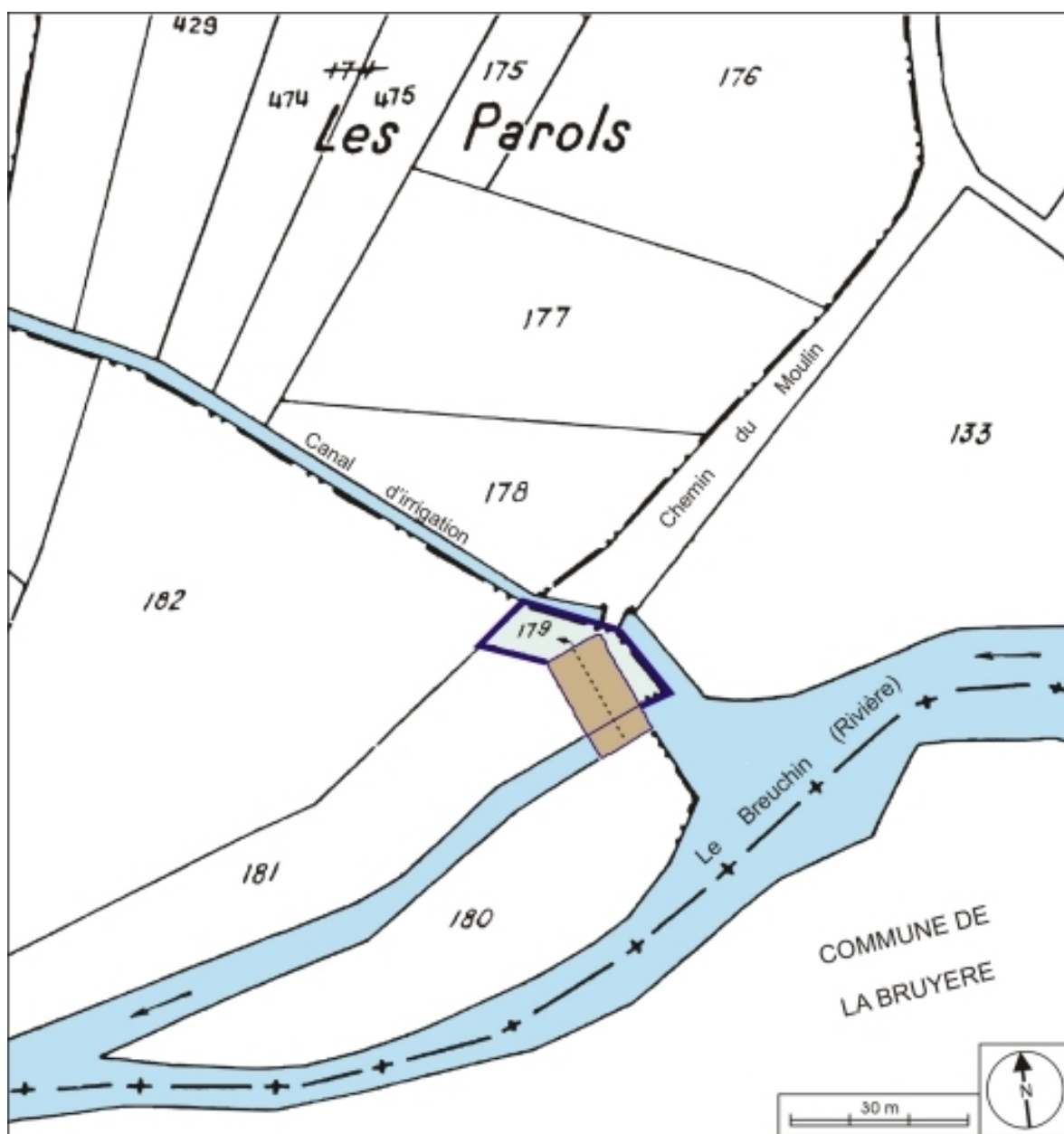
Plan-masse et de situation. Extrait du plan cadastral numérisé, 2005, section B, 1:1000.
