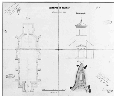
Plan, élévation principale, plan général. Phot. Yves Sancey, Autr. Pourchot (architecte) IVR43_19833900766V
