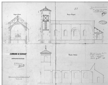
Coupe en travers, coupe en longueur, élévation latérale. Phot. Yves Sancey, Autr. Pourchot (architecte) IVR43_19833900765V
